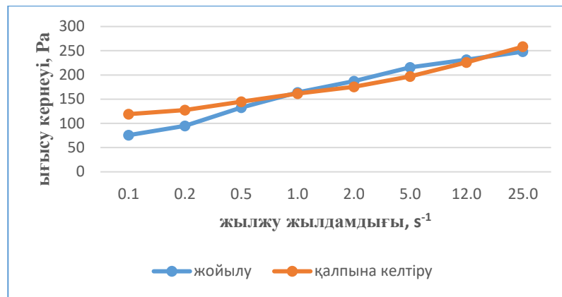
Сурет 22 - Dracoscephalum nutans L. эфир майы мен карбопол негізіндегі гельді зерттеу үлгісі үшін жылжитын ағыстың жылдамдық градиентінің жылжу кернеуінен тәуелділігіндегі гистерезистік эффектілер (1-үлгі)
