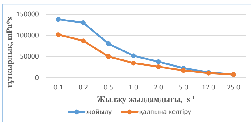
Сурет 19 - Dracoscephalum nutans L. эфир майы мен Na-КМЦ негізіндегі гельдің тиімді тұтқырлығының 20°C температурадағы жылжитын ағысының жылдамдық градиентінен тәуелділігі (7-үлгі)
