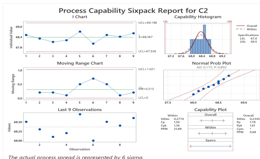
Сурет 45 - Экстрактағы этил спиртінің сандық анықтамасы сапа көрсеткішінің Шухарт бақылау картасы (серия 2)
