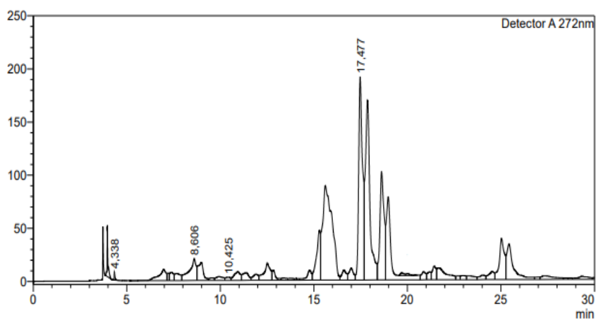
Сурет 20 – Ультрадыбысты экстрактының этилацетатты фракциясының хроматограммасы
