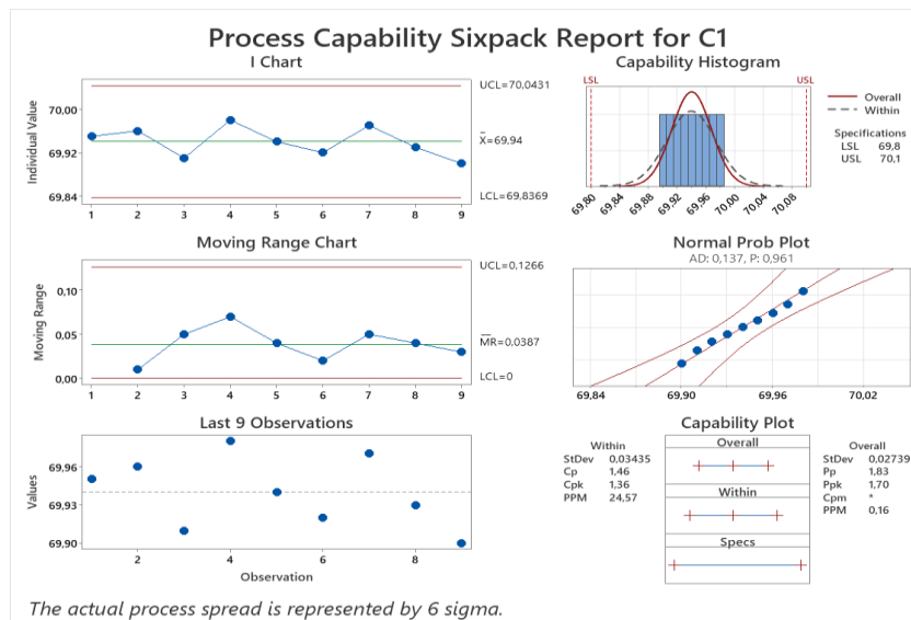
Сурет 29 – Этил спиртінің концентрациясы параметрінің Шухарт бақылау картасы (серия 1)
