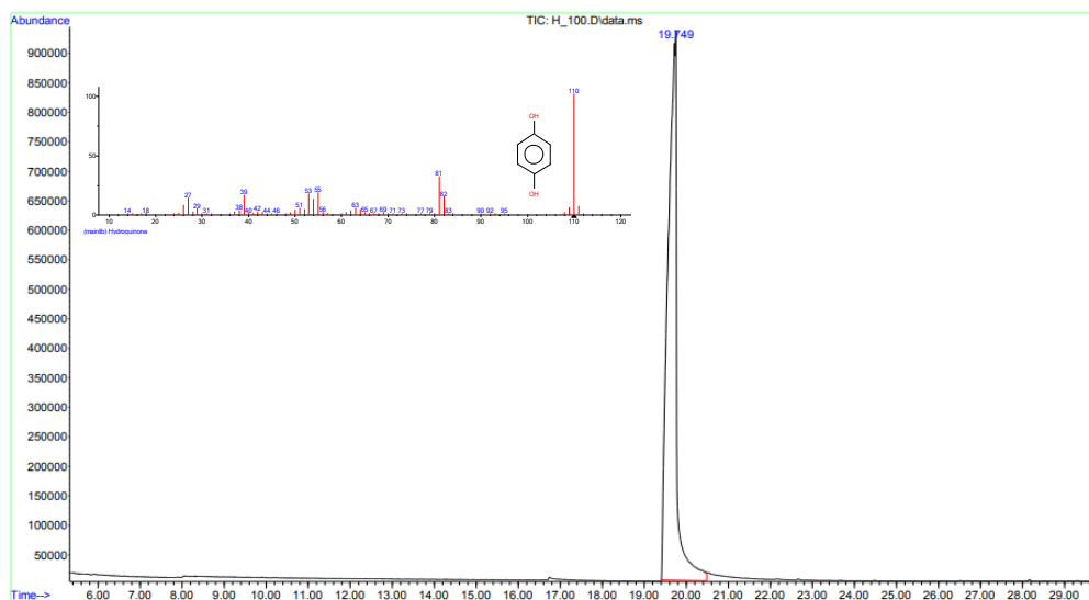
Сурет 24 - СУ Hydroquinone хроматограммасы мен масс-спектрі
