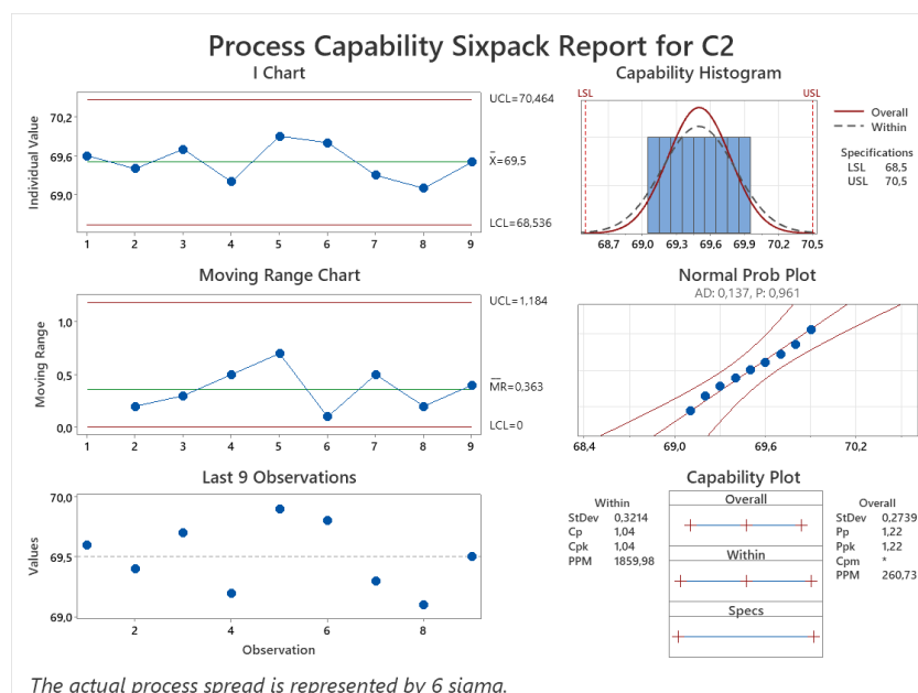
Сурет 36 - Экстрактағы этил спиртiнiң сандық анықтамасы сапа көрсеткішiнiң Шухарт бақылау картасы (серия 2)
