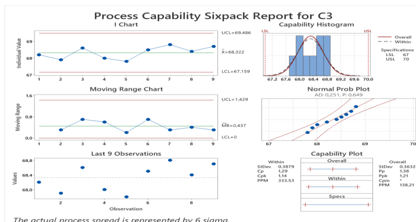
Сурет 46 - Экстрактағы этил спиртінің сандық анықтамасы сапа көрсеткішінің Шухарт бақылау картасы (серия 3)
