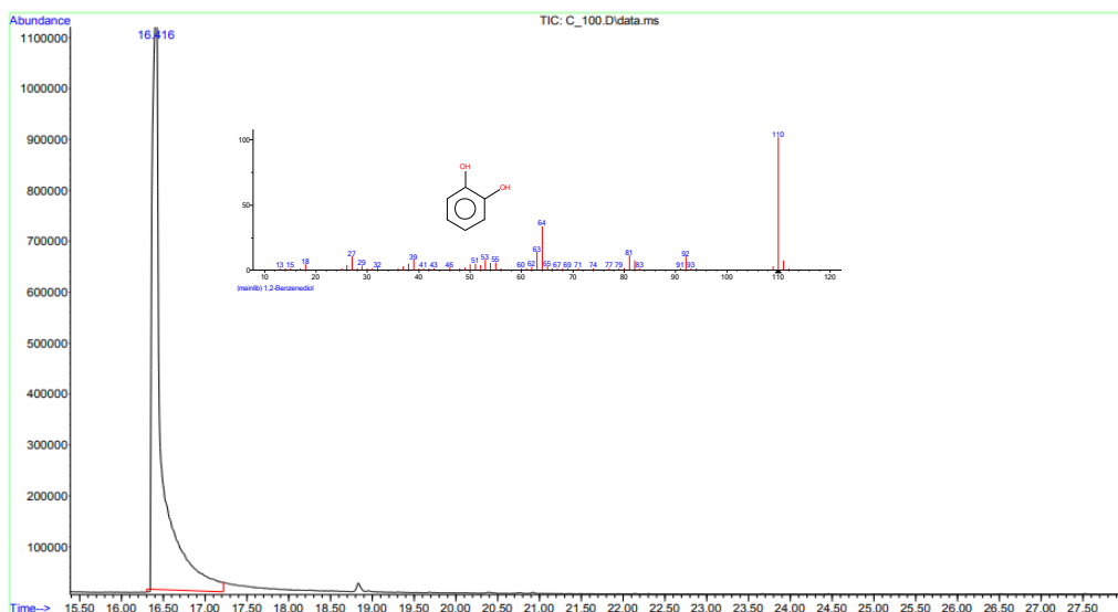
Сурет 23 - СУ Catechol хроматограммасы мен масс-спектрі
