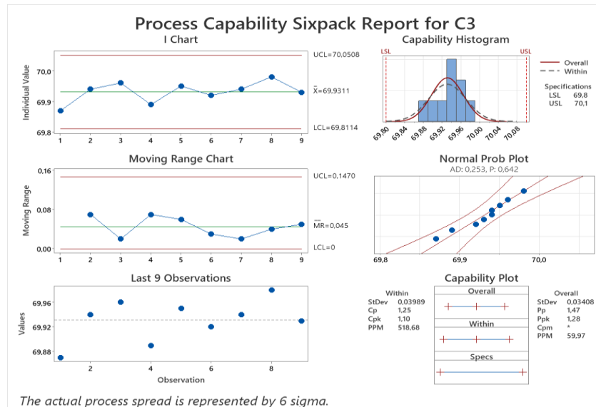
Сурет 31 – Этил спиртінің концентрациясы параметрінің Шухарт бақылау картасы (серия 3)
