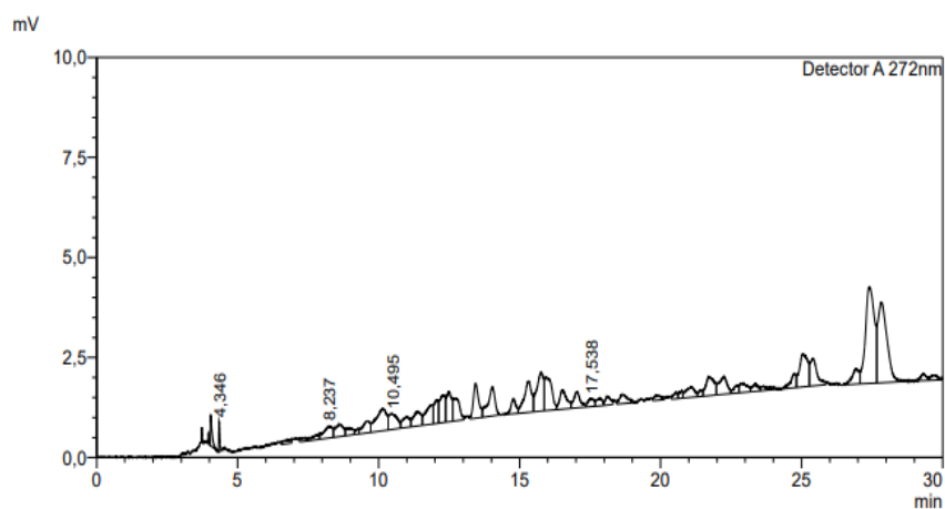
Сурет 21 – Микротолқынды экстрактының дихлорметанды фракциясының хроматограммасы
