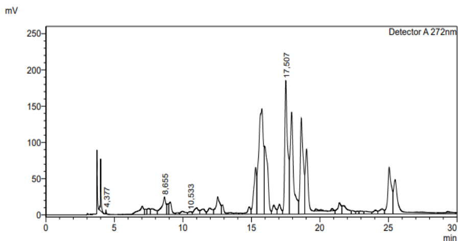
Сурет 19 – Микротолқынды экстрактының этилацетатты фракциясының хроматограммасы
