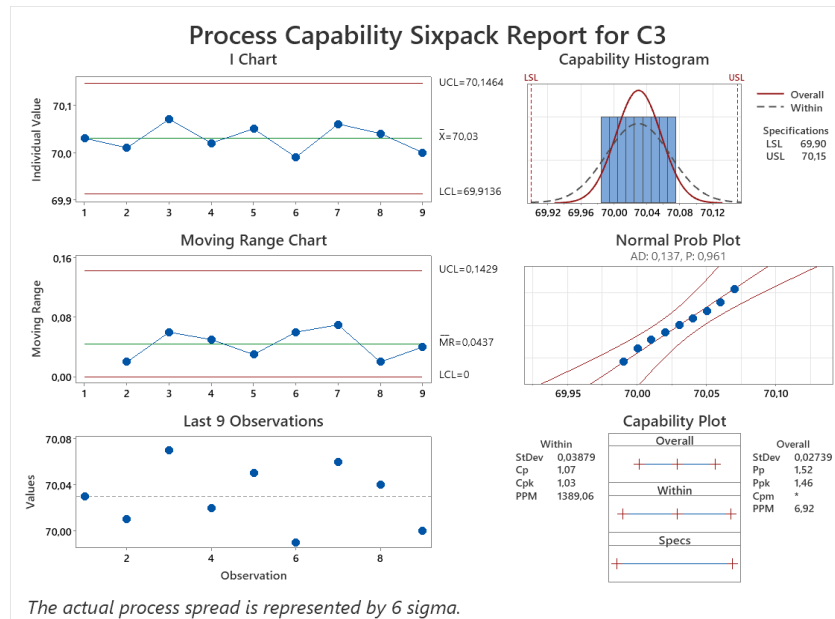
Сурет 40 – Этил спиртінің концентрациясы параметрінің Шухарт бақылау картасы (серия 3)
