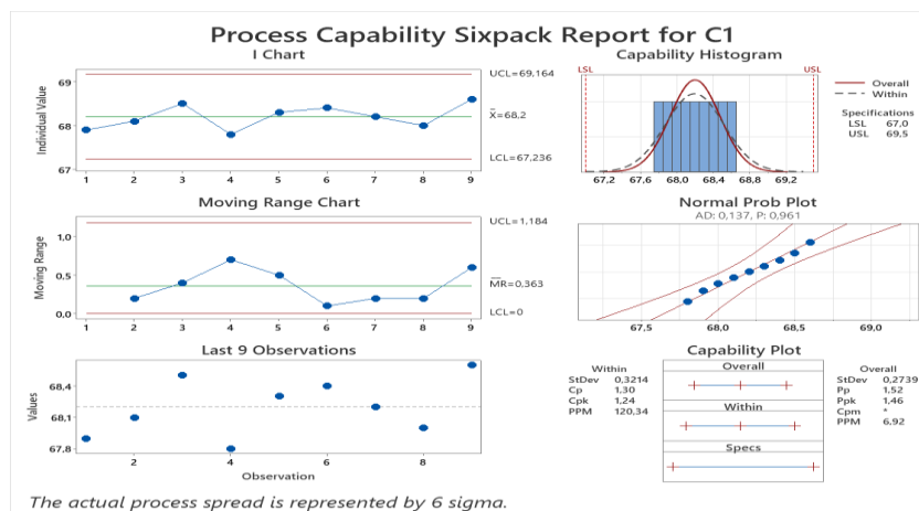
Сурет 44 - Экстрактағы этил спиртінің сандық анықтамасы сапа көрсеткішінің Шухарт бақылау картасы (серия 1)
