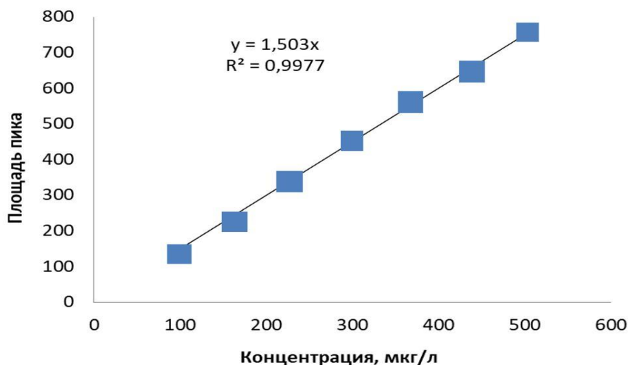
Сурет 26 - Экстрактан алынған Hydroquinone шың аудандарының концентрацияға тәуелділігі
