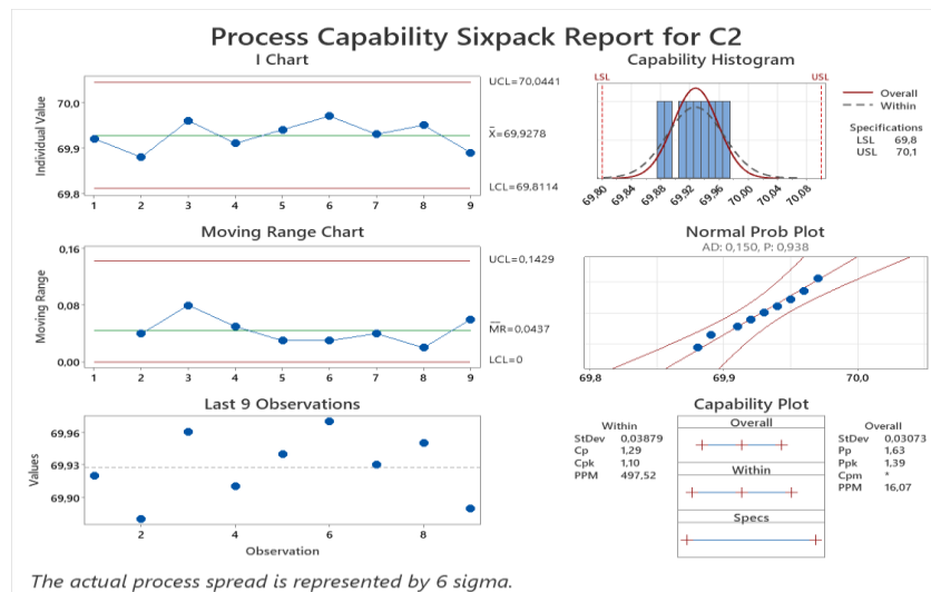
Сурет 39 – Этил спиртінің концентрациясы параметрінің Шухарт бақылау картасы (серия 2)
