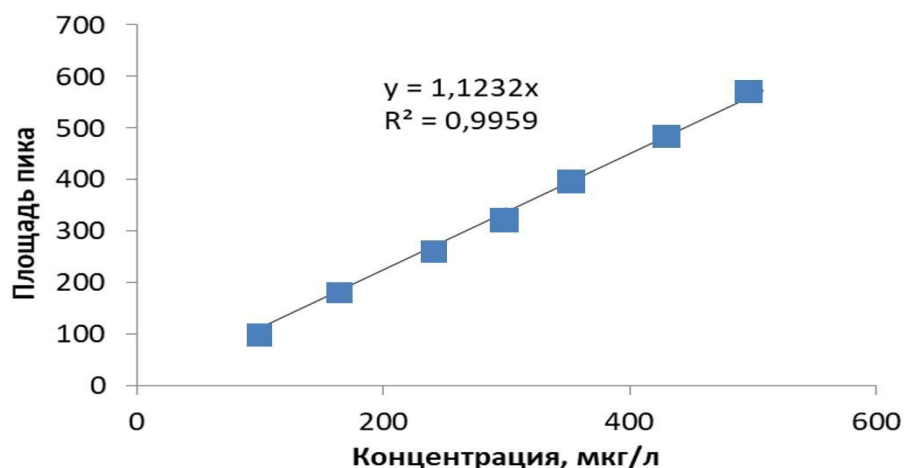
Сурет 25 - Экстрактан алынған Catechol шың аудандарының концентрацияға тәуелділігі
