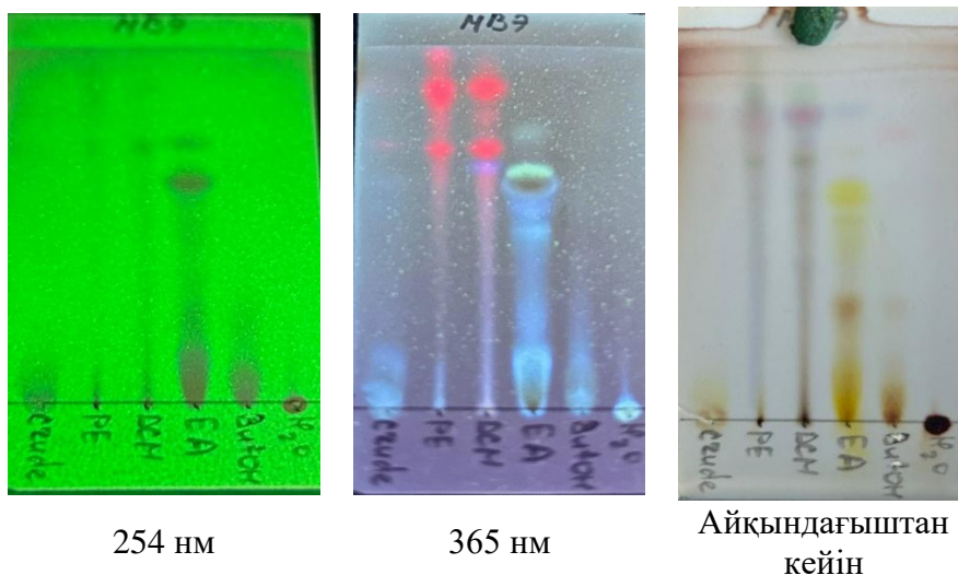
Сурет 16 - Микротолқынды экстракцияның жылжымалы фазадағы фракциясы
