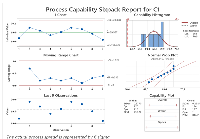
Сурет 35 - Экстрактағы этил спиртiнiң сандық анықтамасы сапа көрсеткішiнiң Шухарт бақылау картасы (серия 1)
