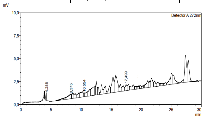
Сурет 22 – Ультрадыбысты экстрактының дихлорметанды фракциясының хроматограммасы
