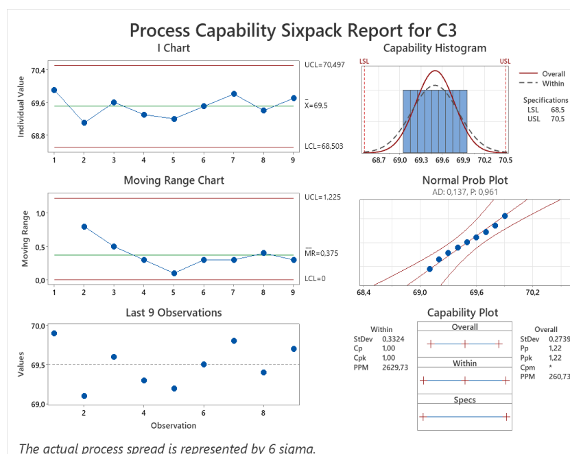
Сурет 37 - Экстрактағы этил спиртінің сандық анықтамасы сапа көрсеткішінің Шухарт бақылау картасы (серия 3)
