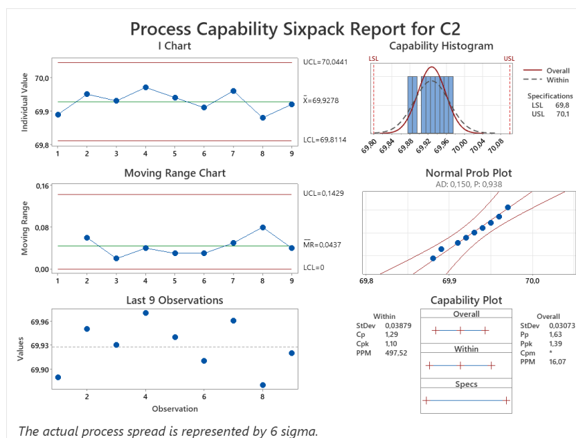
Сурет 30 – Этил спиртінің концентрациясы параметрінің Шухарт бақылау картасы (серия 2)
