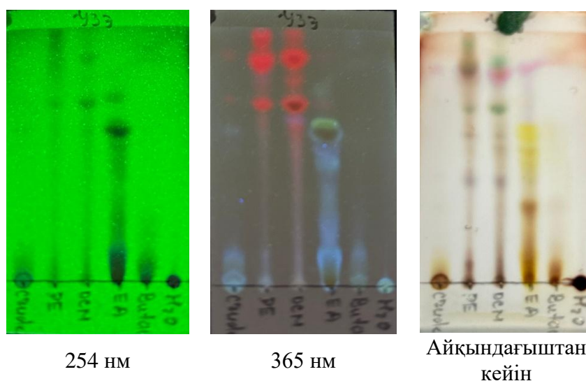
Сурет 17 - Ультрадыбысты экстракцияның жылжымалы фазадағы фракциясы
