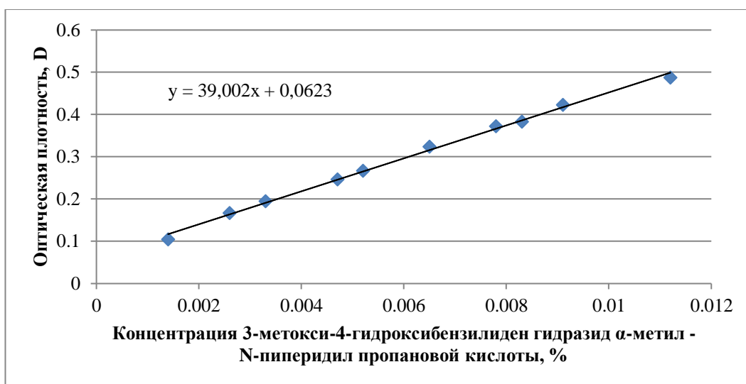
Рисунок 38 – График и уравнение линейной зависимости УФ-спектрофотометрического определения 3-метокси-4-гидроксибензилиденгидразид α-метил-β-(N-пиперидил)пропановой кислоты
