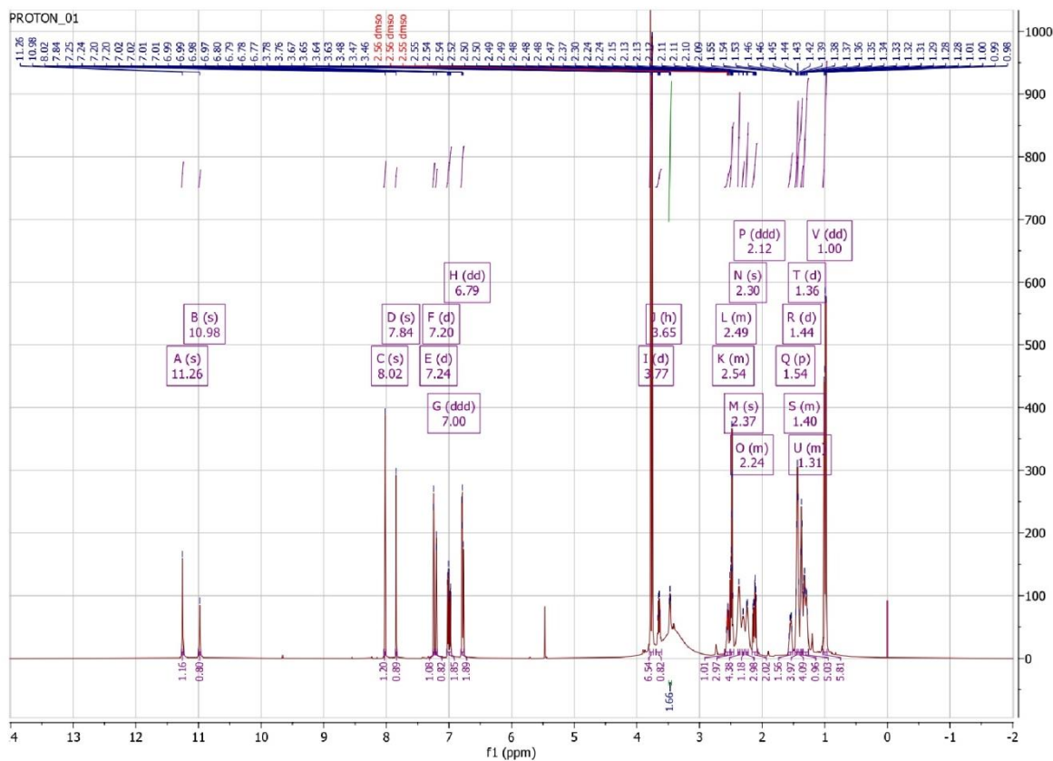
Рисунок Д.1 – ^1\text{H} ЯМР-спектр 3-метокси-4-гидроксibenзилиден гидразид \alpha -метил- \beta -( N -пиперидил)пропановой кислоты
