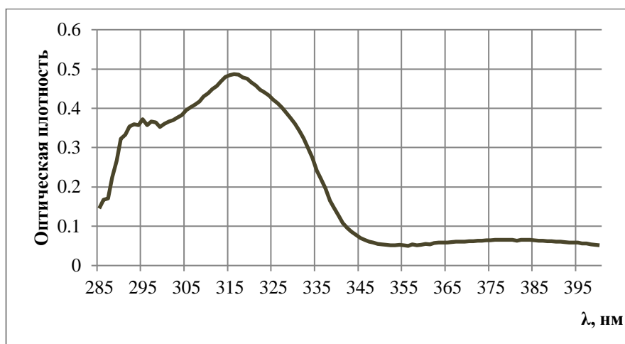
Рисунок 37 – УФ-спектр 0,01 % раствора 3-метокси-4-гидроксибензилиденгидразида \alpha -метил- \beta -( N -пиперидил)пропановой кислоты в этаноле
