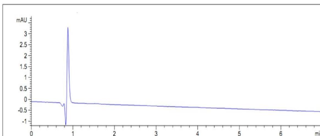
Рисунок 34 – Хроматограмма бланк-раствора
