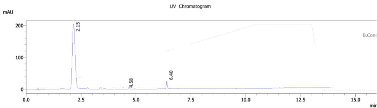
Рисунок 35 – Хроматограмма испытуемого раствора 3-метокси-4-гидроксипиперидилпропановой кислоты \alpha -метил- \beta -( N -пиперидил)пропановой кислоты
