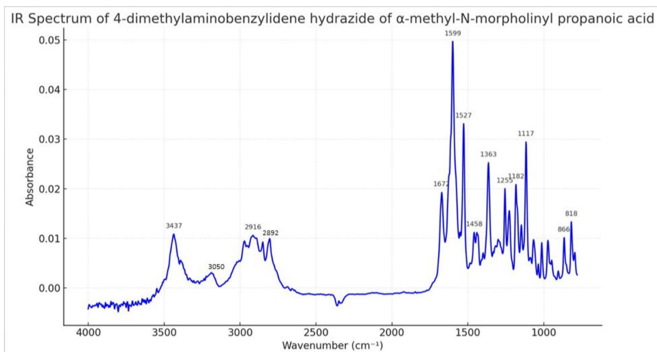
Рисунок 29 – ИК-спектр 4-диметиламинобензилиденгидразид \alpha -метил- \beta -( N -морфолил)пропановой кислоты
