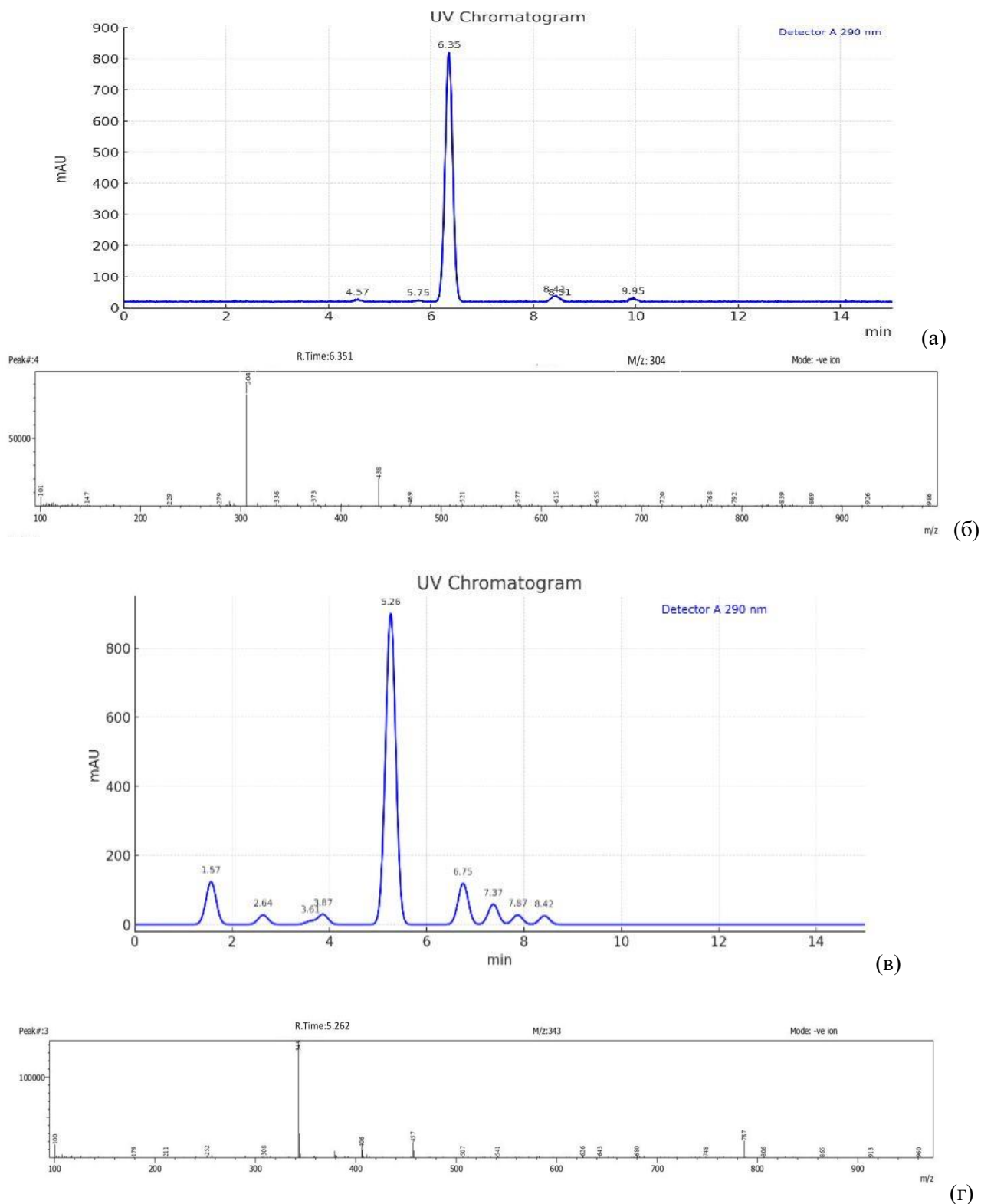
Рисунок 22 – ВЭЖХ–УФ хроматограммы и масс-спектры 3,4-дигидроксибензилиденгидразид \alpha -метил- \beta -( N -пиперидил)пропановой кислоты (а-б) с концентрацией 0,001 г/мл, 3,4-дигидроксибензилиденгидразид \alpha -метил- \beta -( N -морфолил)пропановой кислоты (в-г) с концентрацией 0,001 г/мл
