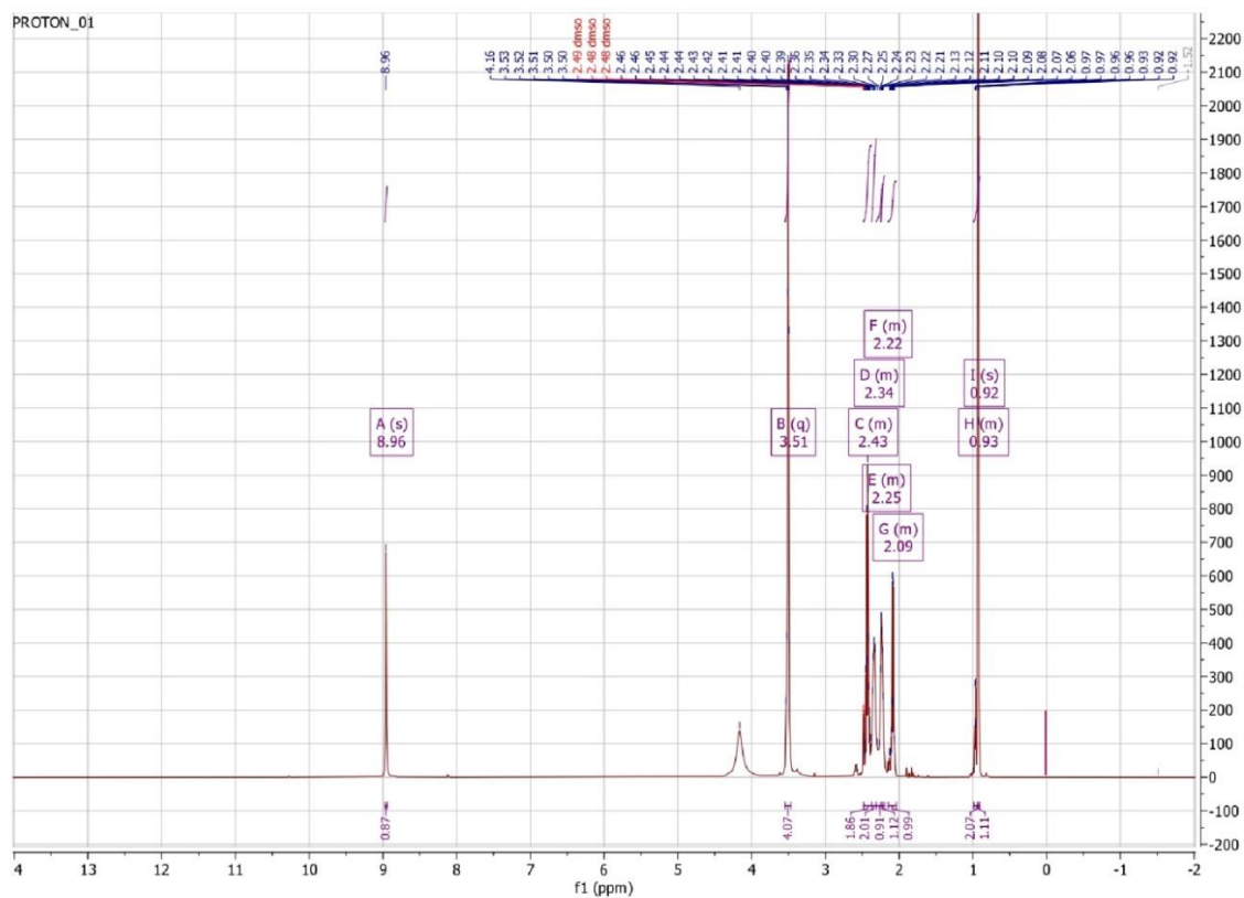
Рисунок Д.2 – ^1\text{H} ЯМР-спектры 1.4 - 4-диметиламинобензалиден гидразид \alpha -метил- \beta -( N -пиперидил)пропановой кислоты; 2.2 – гидразид \alpha -метил- \beta -( N -морфолил) пропановой кислоты
